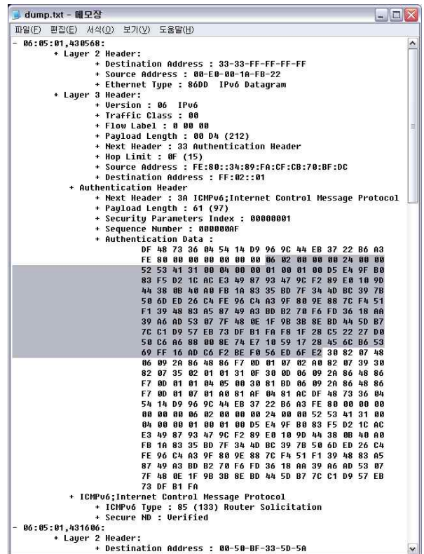
그림 5. Secure ND 메시지 검증정보
