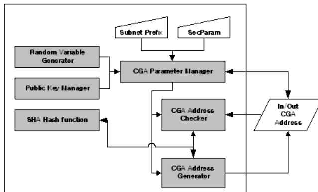
그림 1 CGA 모듈 블럭다이어그램 Fig. 1. CGA Module Block Diagram
