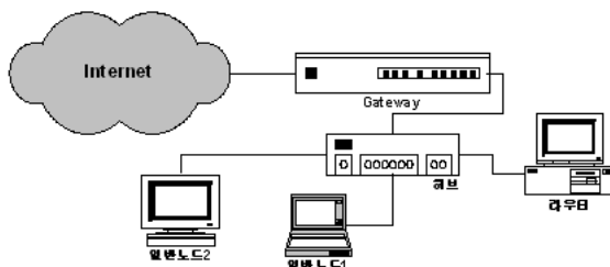
그림 3 테스트를 위한 link local 네트워크 Fig. 3. Link local network for testing modules
